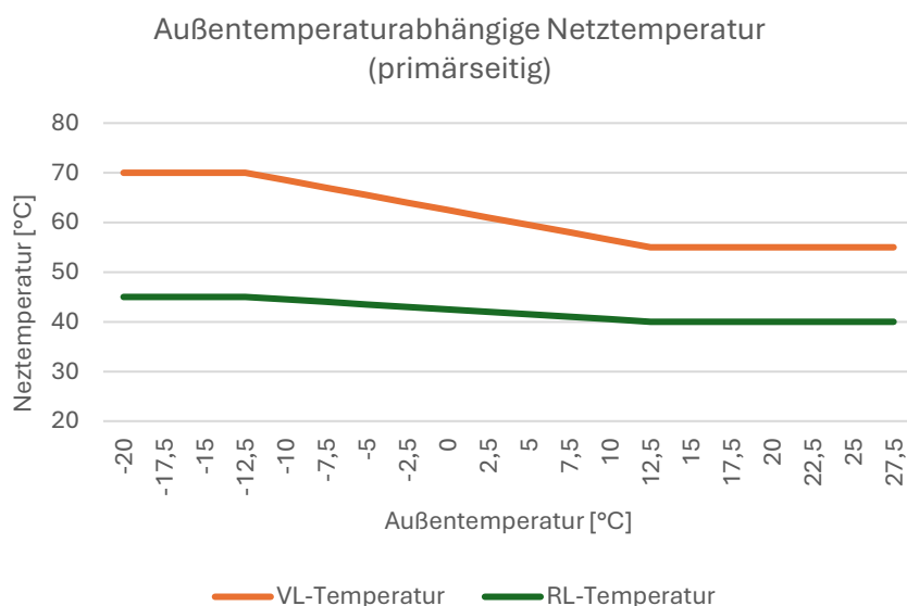
Abbildung 2: Wärmenetztemperaturen
