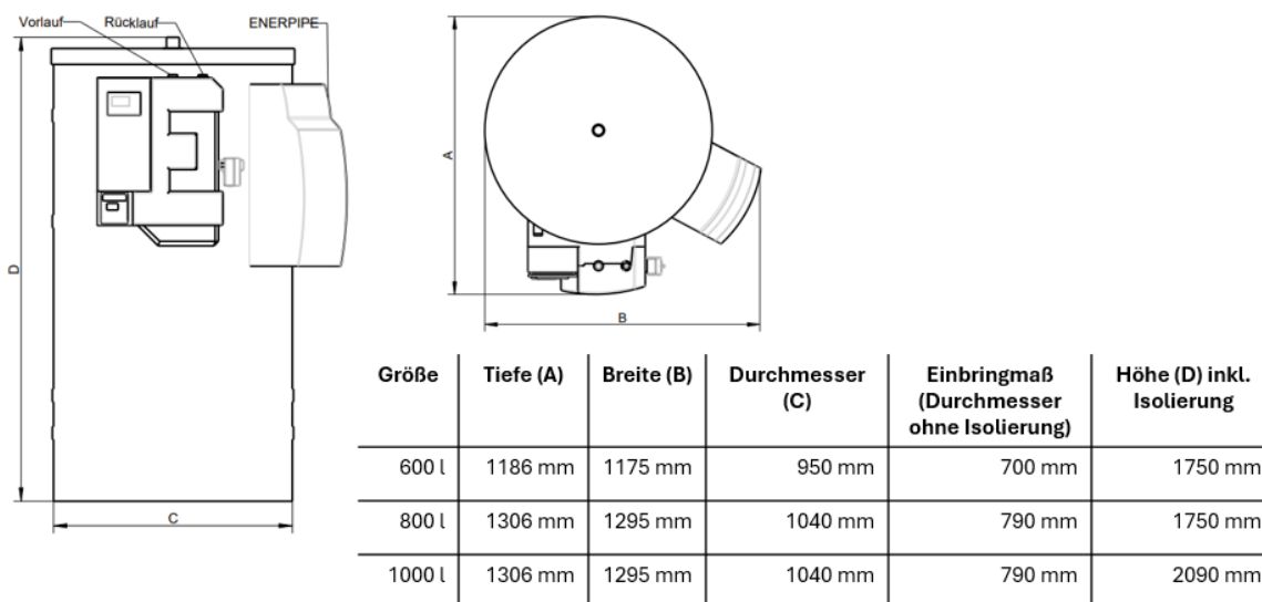
Abbildung 3: Aufstellmaße (Enerpipe)
